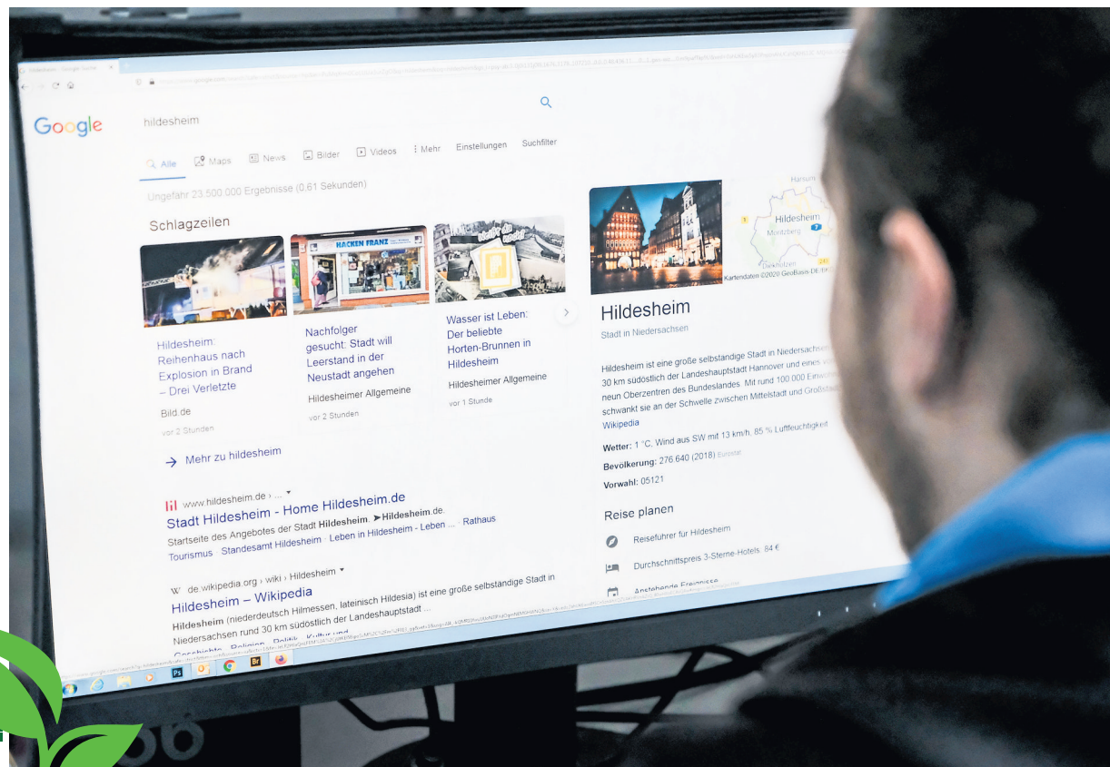
23,5 Millionen Treffer bei der Suche nach dem Stichwort „Hildesheim“: Sie werden von gigantischen Rechenzentren serviert, die viel Strom verbrauchen. Der Verbrauch der Endgeräte kommt noch dazu.
